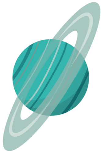
URANUS
