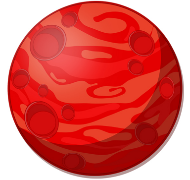
MARS
