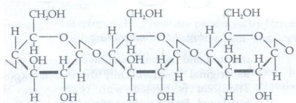
Fig. 2.26: Cellulose
