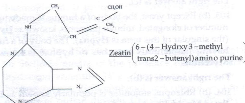
Fig. 3.20: Zeatin
