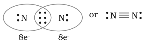
N_2 molecule
