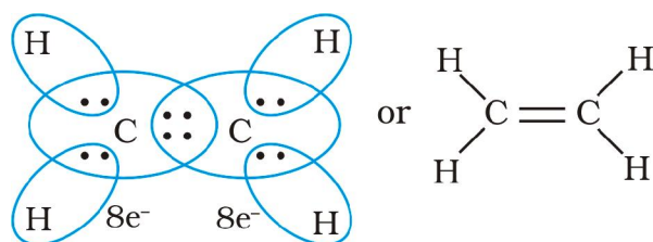
C_2H_6 molecule
