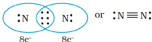
N_2 molecule
