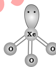
(e) Pyramidal
