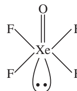
\text{XeOF}_4
