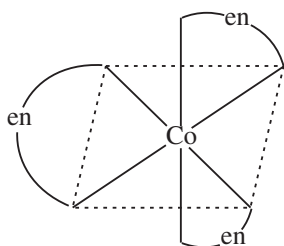
d -Tris-(ethane-1,2-diamine) cobalt (III)
